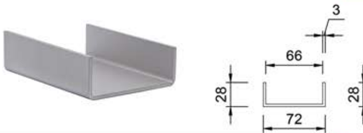
BALKO Stoß-Verbinder 70 mm
