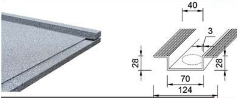
Fräsung für Alurinne
